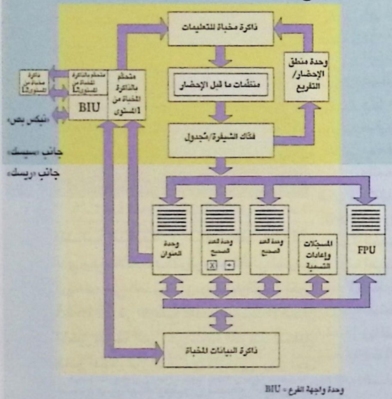
وحدة واجهة الفروع - BIU من المحتمل أن تتخذ هيكلية الجيل المبكر من Nx586. الموضحة هنا، إلى Nx686.
