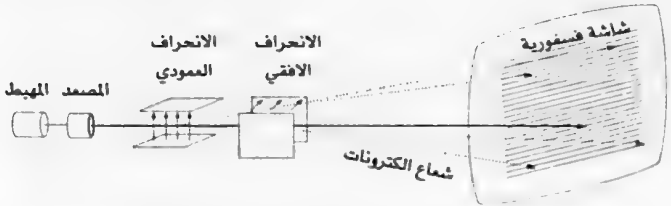
رسم توضيحي لتقنية انبواب الاشعة المهبطية CRT
