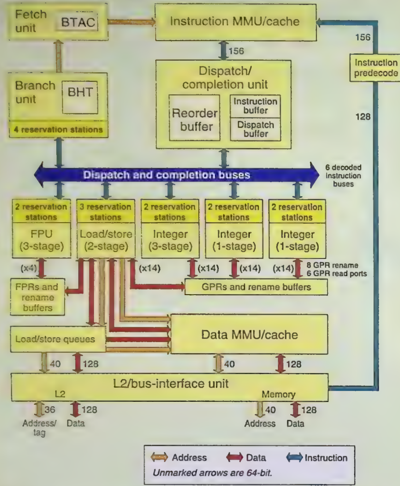
شكل تخطيطي لمعالج «باور بي سي 620». ورغم شبيهه الكبير مع تركيب معالج «باور بي سي 604»، فإنه يختلف عنه من حيث أن وحدات GPR، FPR والنوازل الداخلية بعرض 64 بت، وتأتي وحدات الحل المسبق للشيفرة قبل ناكرة الشيفرة مما يساعد على اختصار خط العمليات للمعالج إلى مرحلة واحدة.
