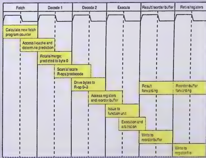
إن مراحل الناقل في K5 تعطي دليلاً إضافياً على طبيعته الشبيهة بـ «ريسك». إن K5 وحدة تنفيذ لتحميل وتخزين العمليات. كما أنه يضيف مرحلة ما قبل إرسال النتائج للبرنامج والتي تتم فيها إعادة سلسلة العمليات.
